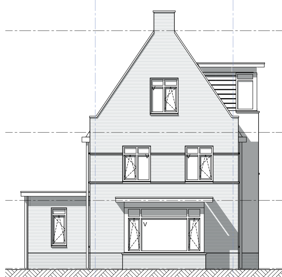
Linkergevel
