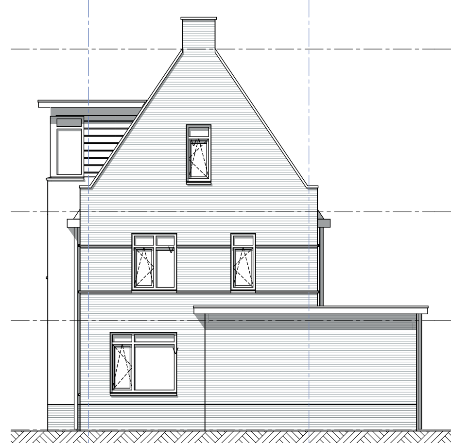
Rechtergevel
