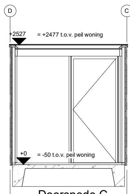
Doorsnede C
