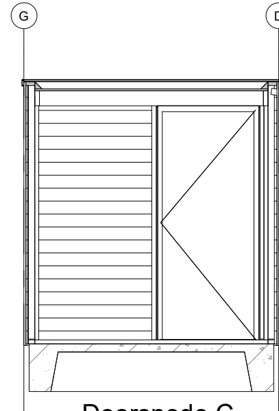
Doorsnede C
