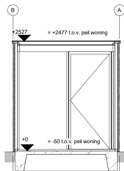
Doorsnede A
