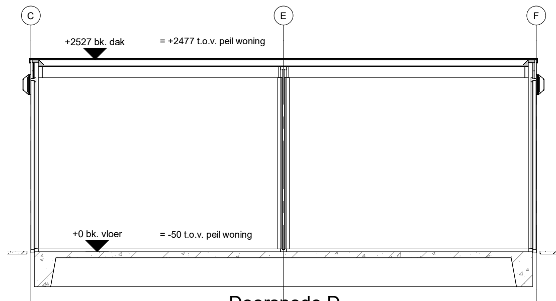
Doorsnede D
