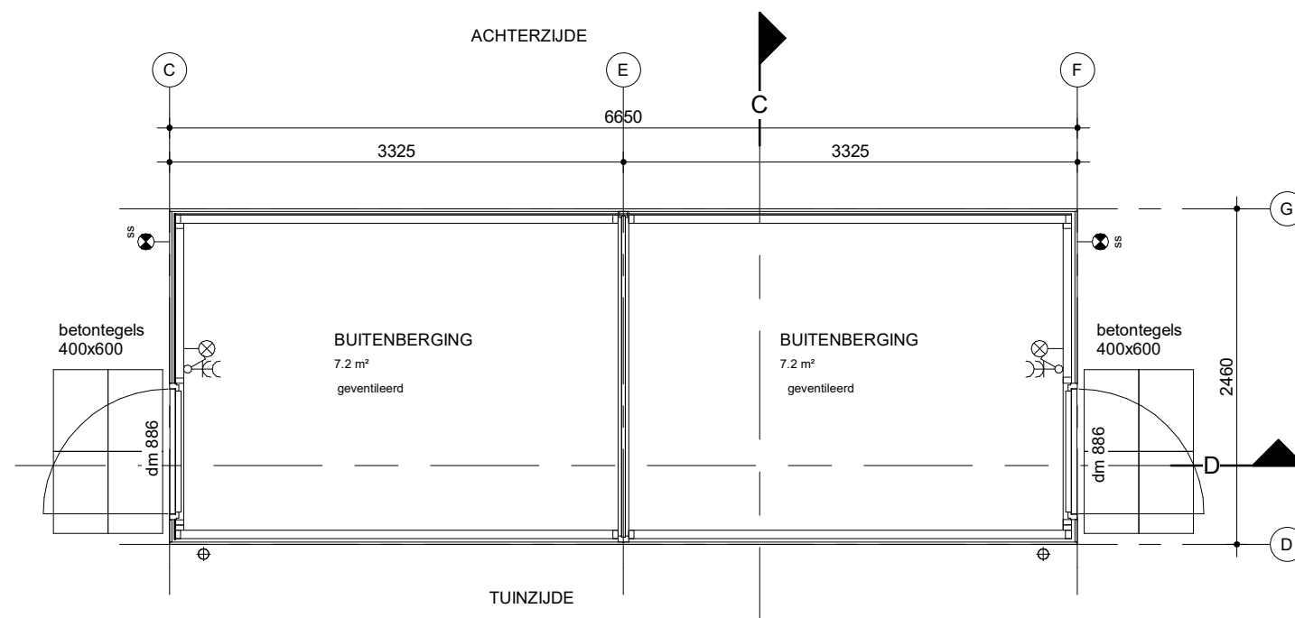
Begane grond
