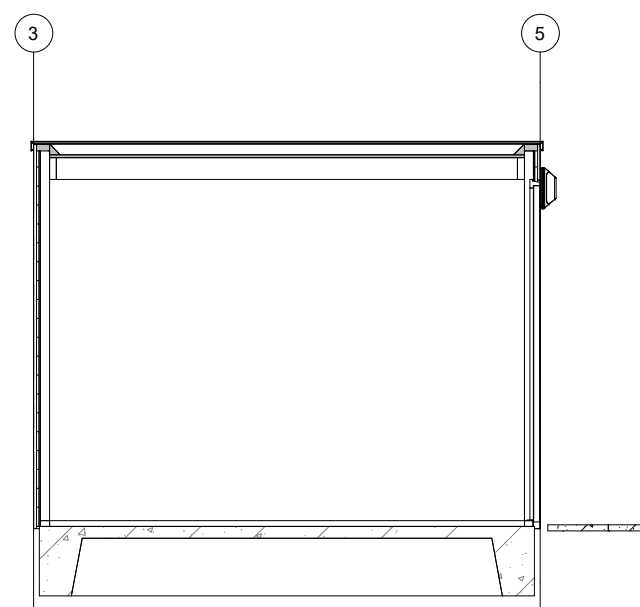
Doorsnede D
