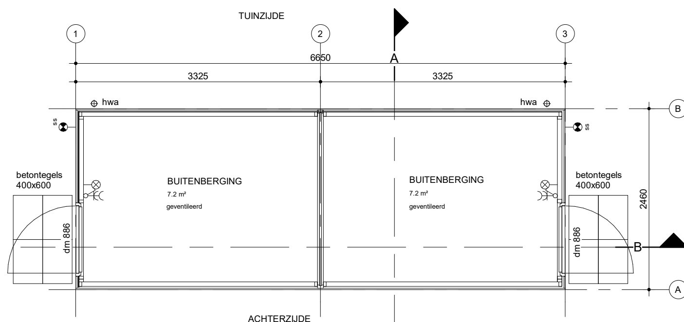
Begane grond
